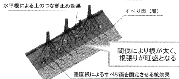
根系の引き抜き抵抗力模式図 (北原：2006を改変)
